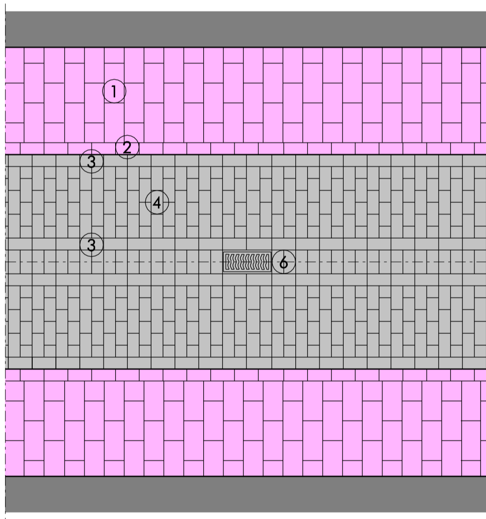
DETALLE DE PAVIMENTACION 1 CALLE CHAPINERIA
