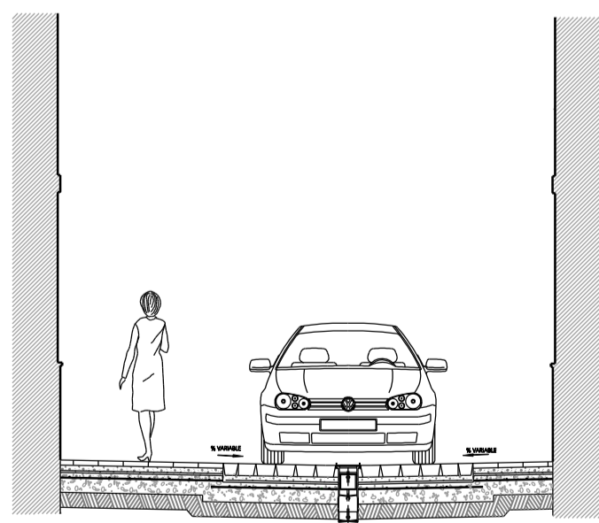
SECCION TIPO POR CALLE
