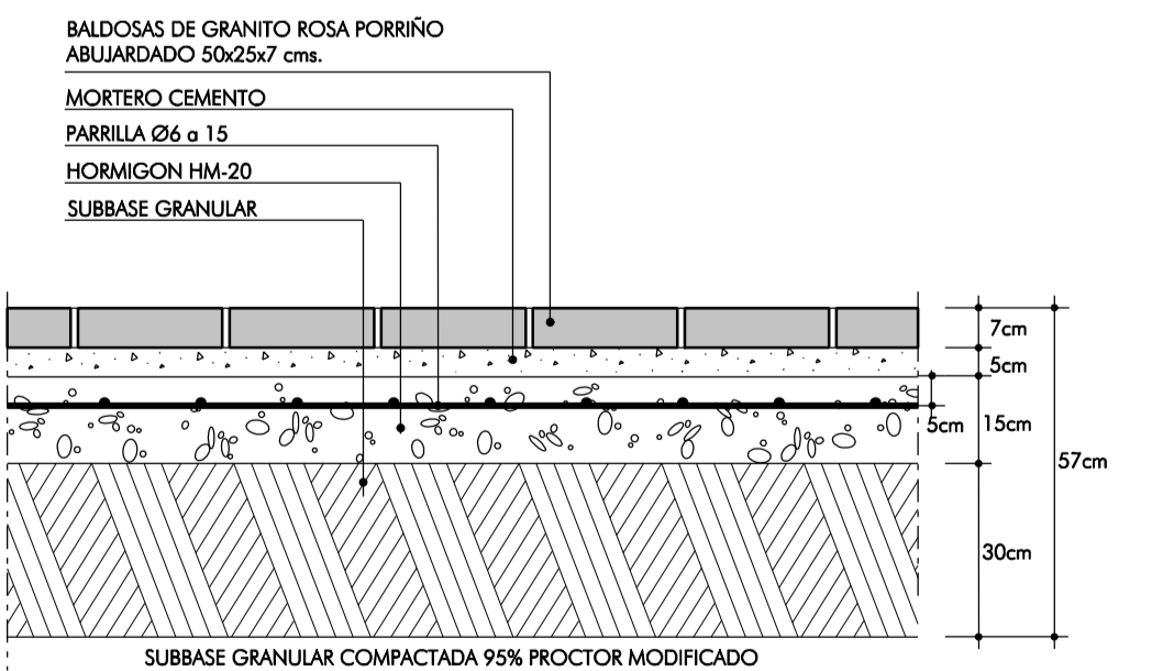
DETALLE DE PAVIMENTACION ESCALA 1:15
