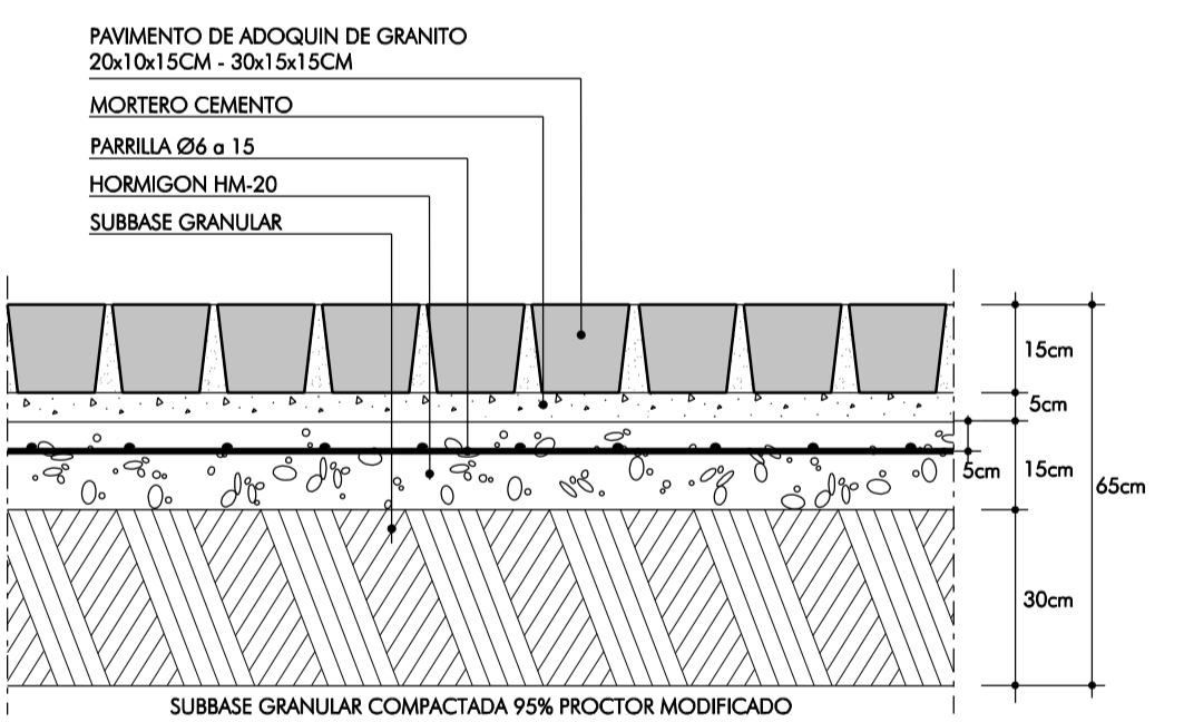
DETALLE DE PAVIMENTACION (ZONA RODADA CON ADOQUIN) ESCALA 1:15
