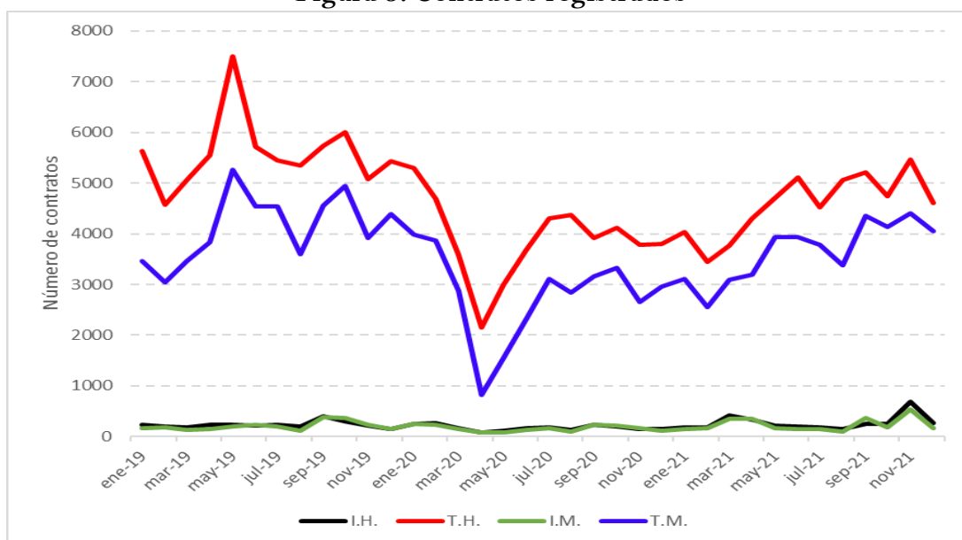
Figura 5. Contratos registrados
